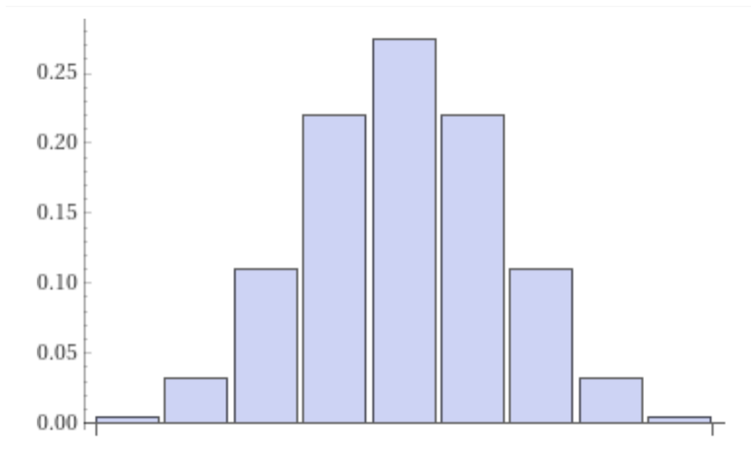
Figure 58: Densità binomiale B(8, \frac{1}{2}) . I possibili valori della variabile aleatoria sono 0, \dots, 8 e il più probabile è 4. Screenshot da WolframAlpha.
