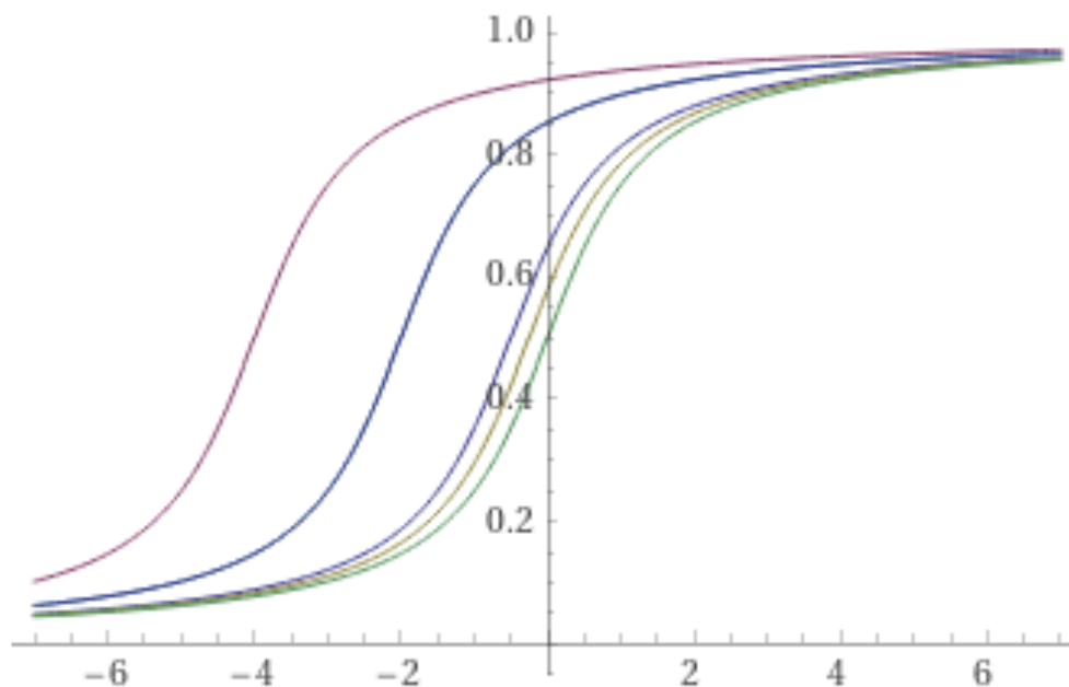
Figure 56: Verde: funzione di ripartizione di una certa v.a. X ; altri colori, dall'alto verso il basso: funzioni di ripartizione di X_1, X_2, X_3, X_4 ; non sono rappresentati gli infiniti grafici delle funzioni di ripartizione di X_5, X_6, \dots ma li si immagini sempre più prossimi alla curva in verde, realizzando la convergenza in legge di X_n a X . Screenshot da WolframAlpha.
