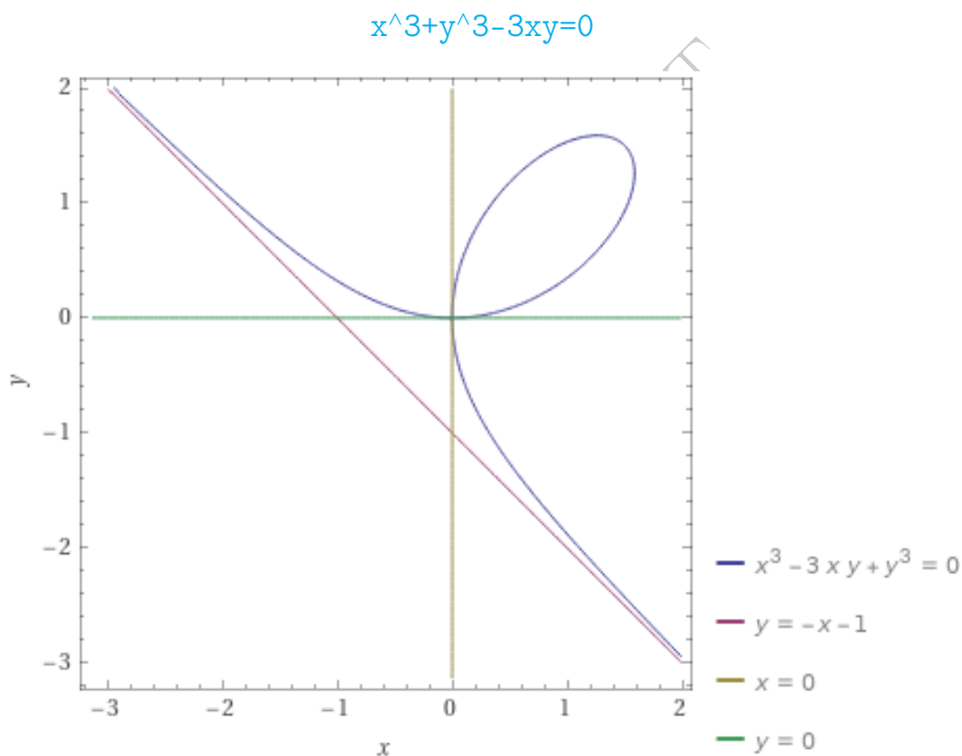
Figure 13: Folium di Cartesio e suo asintoto y = -x - 1
