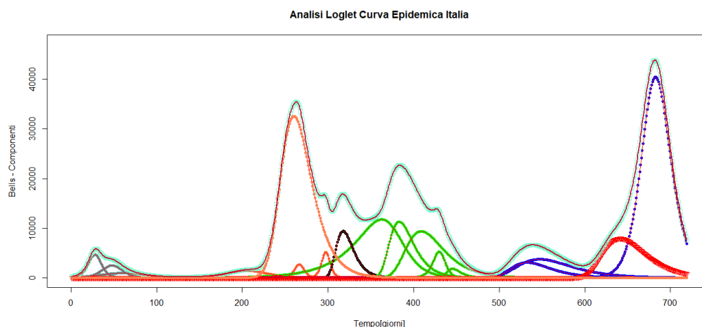
Figure 65: Loglet per contagi SARS-CoV-2, 2020-2021. By Carlo Del Vecchio.
